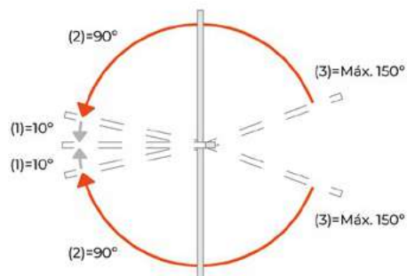
Nota: (1) Corsa finale, (2) Velocità di chiusura, (3) Velocità di apertura massima
